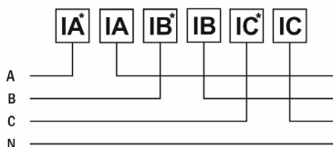
Рис. 5 – Подключение напрямую
