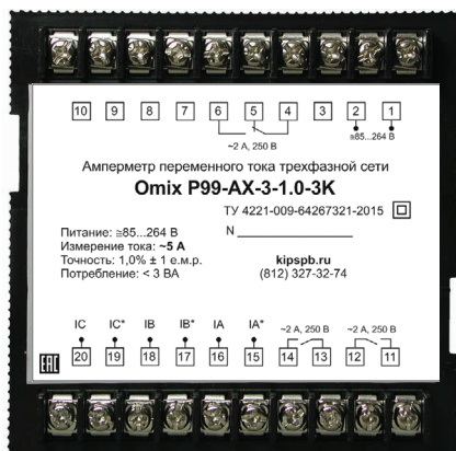
Рис. 7 – Задняя панель прибора
