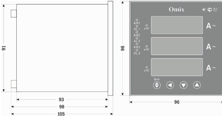
Рис. 3 – Размеры прибора
